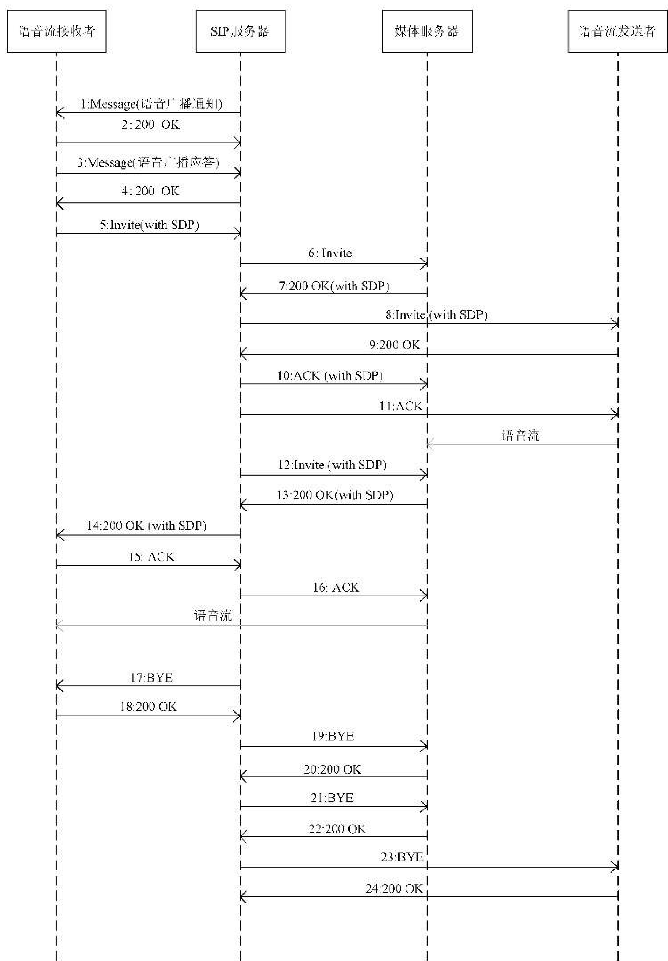
图 27 SIP 服务器发起广播流程
