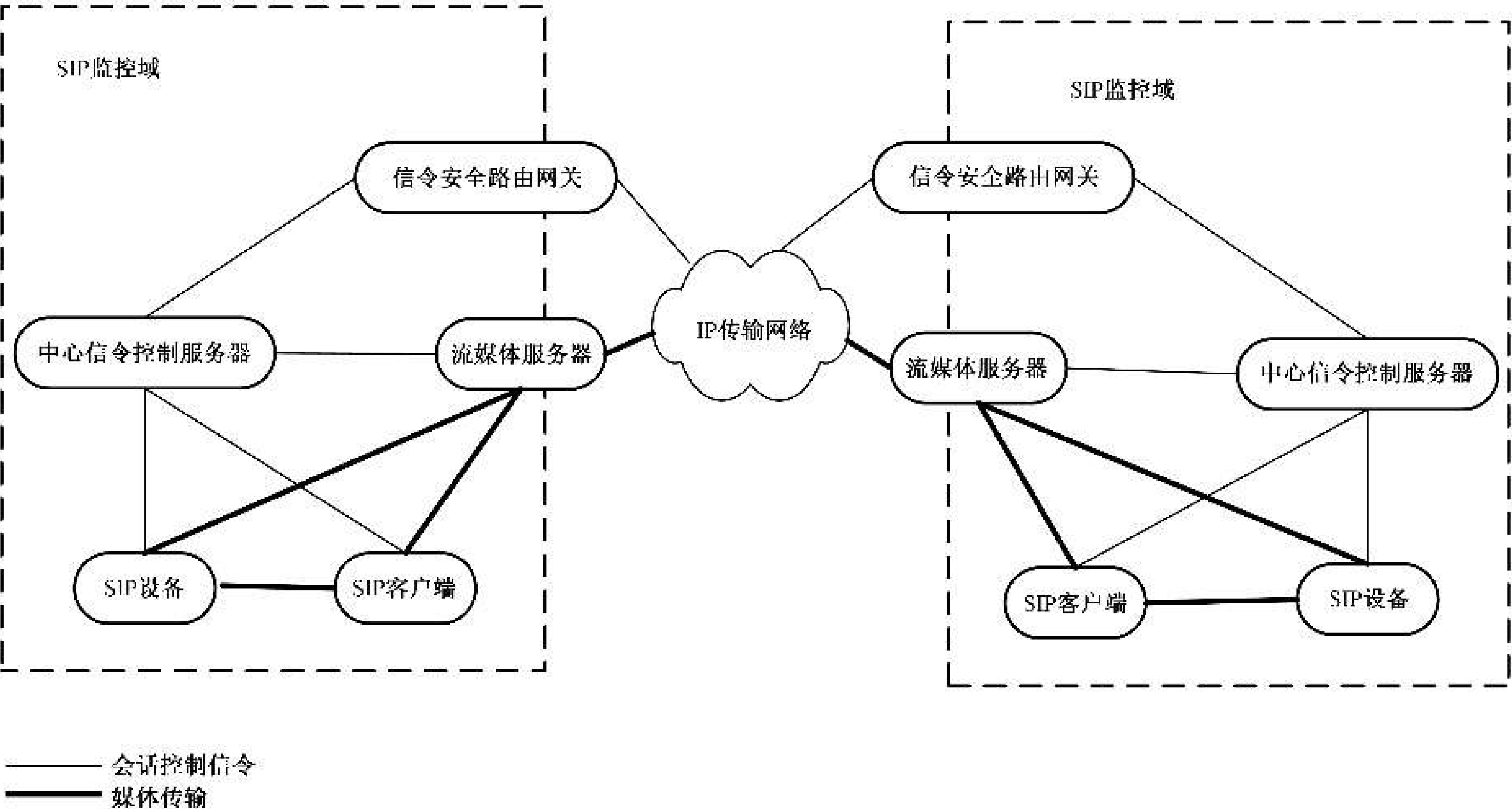
图 1 SIP 监控域互联结构示意图
