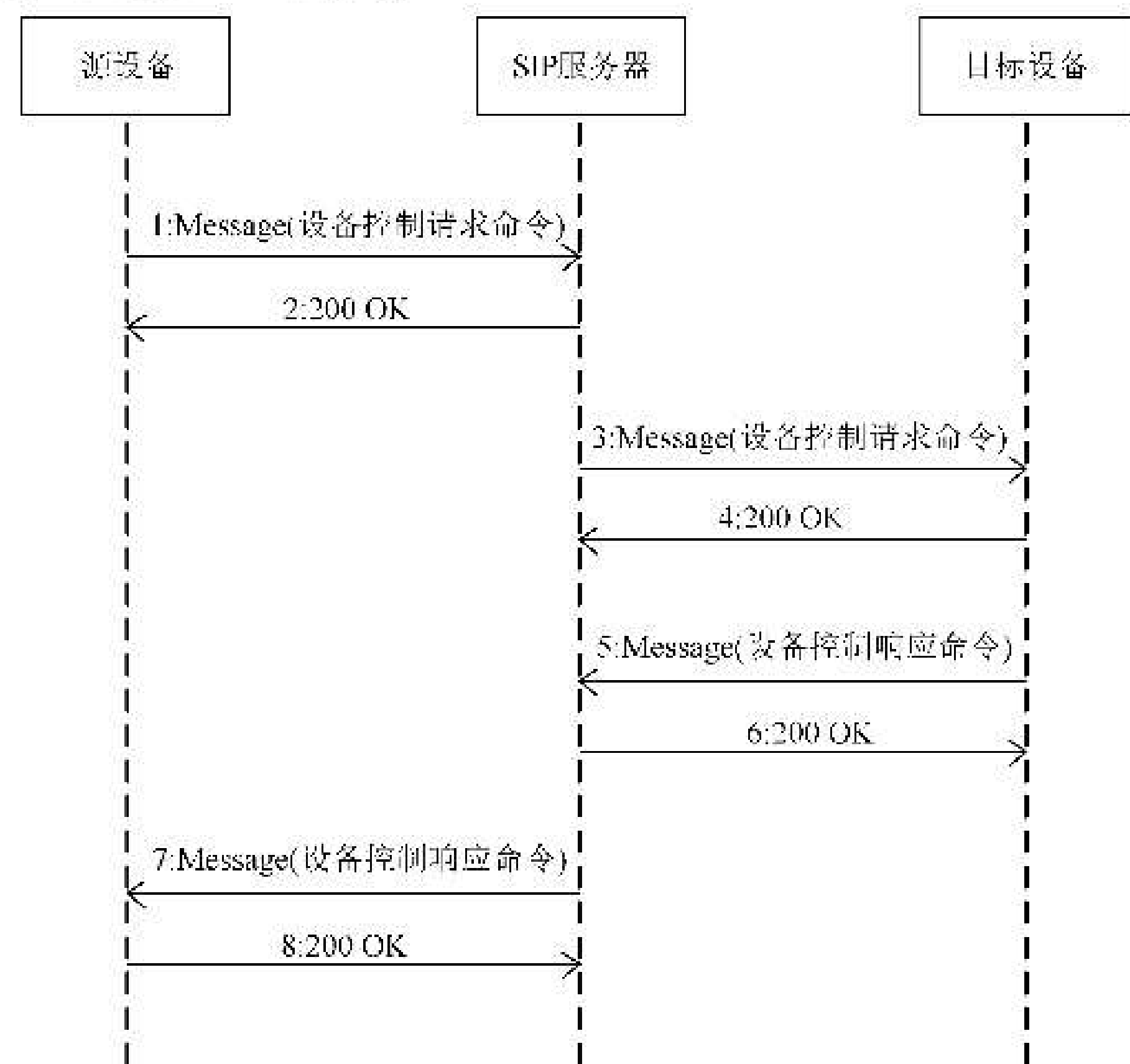
图 14 有应答设备控制流程
